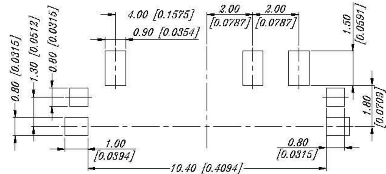
P.C.B LAYOUT
