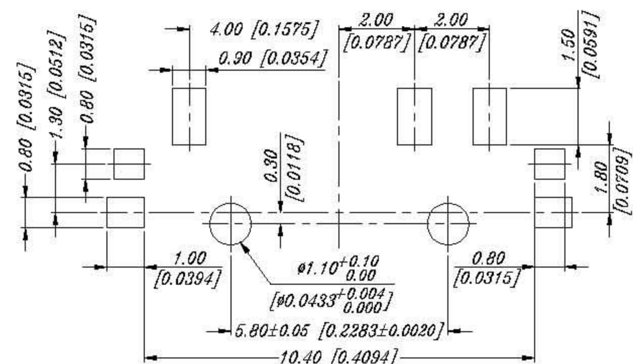
P.C.B LAYOUT
